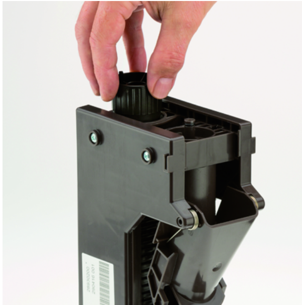
Abb. 31: Brüheinheit Gewinde lösen
