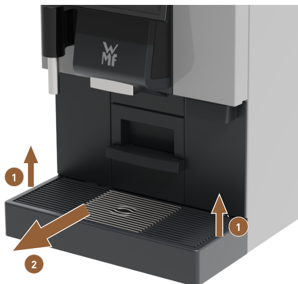
Abb. 37: Tropfschale entnehmen
